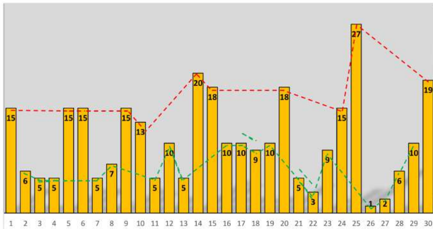
• شکل ۱- عمر انباشت باطله‌های معدنی و فراوری استان (خط سبز دارای عمر زیر میانگین و خط قرمز دارای عمر بالای میانگین)
