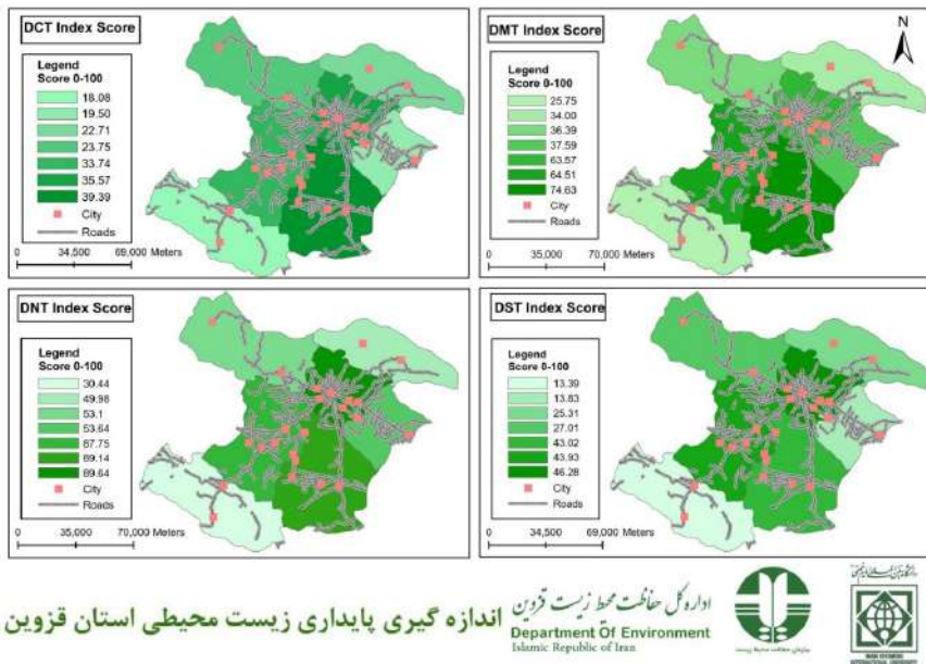
• شکل ۳- شاخص‌های ارزیابی پایداری محیط زیستی در پهنه‌های آمایشی استان قزوین (DNT, DST, DMT, DCT)
