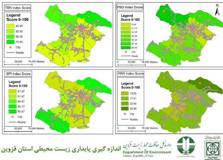
• شکل ۲- شاخص‌های ارزیابی پایداری محیط زیستی در پهنه‌های آمایشی استان قزوین (TBN, PBD, SPI, PAR)
